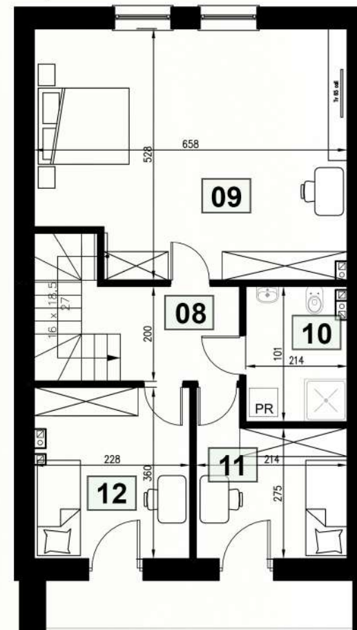
PIĘTRO
